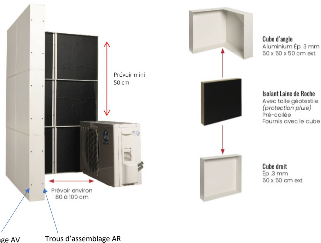
Installation de l'isolant (étape 4)
